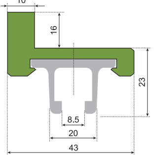
CG - AL - 615B
