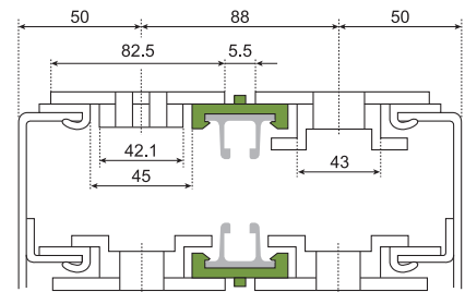
CG - AL - 615B
